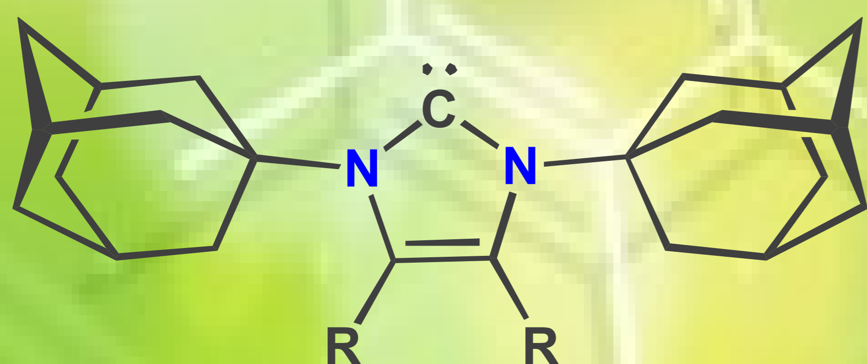
Diadamantyl-NHC Arduengo 1991
