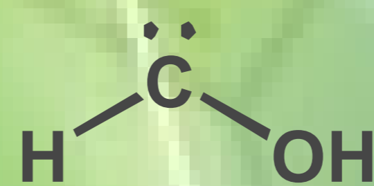
Hydroxycarbene Schreiner, Reisenauer 2008
